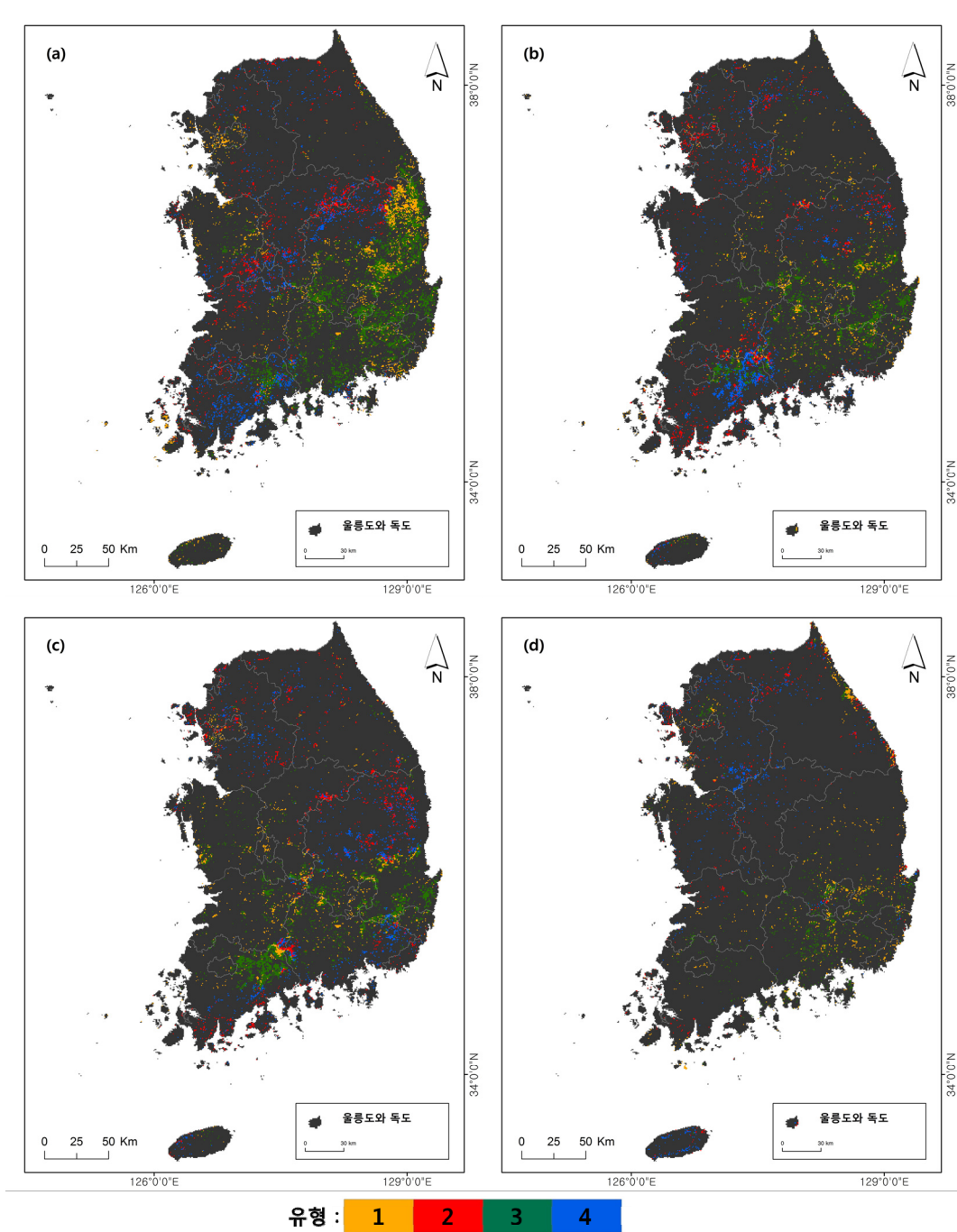
그림 6. 5월 NDVI와 SPI별 변동계수 상관관계 유형 분류(95% 유의수준 만족)
