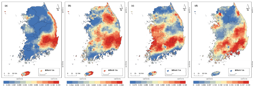
그림 4. 2000~2014년 5월 SPI 변동계수(%)
