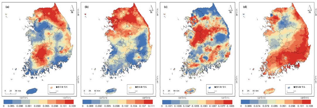
그림 3. 2000~2014년 3월 SPI 변동계수(%)
