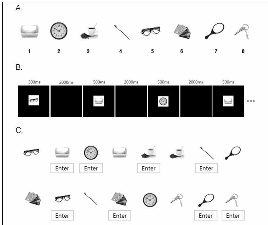
그림 1. 계열적 행동 조절 과제: A는 계열 내 요소 8개를 차례대로 나타낸 것이고, B는 과제의 진행 방식을 나타낸 것이다. 자극은 500ms동안 화면에 제시되며, 자극 간 간격은 2000ms이다. C는 자극이 제시되는 순서와 그에 따른 정반응(Enter)의 예를 나타낸 것이다. Enter 표시의 순서는 계열의 순서와 동일하다.
