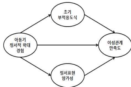
그림 2. 경쟁모형
