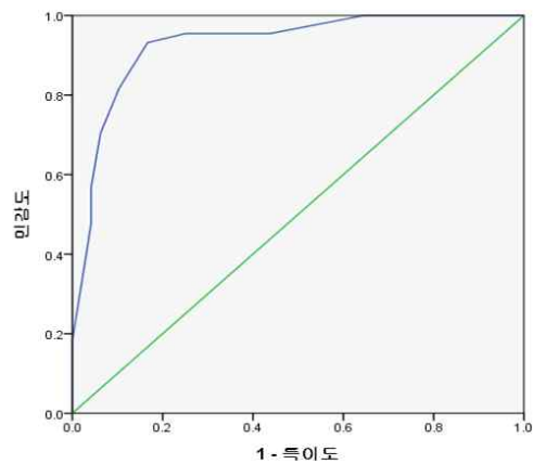
그림 2. ROC 곡선
