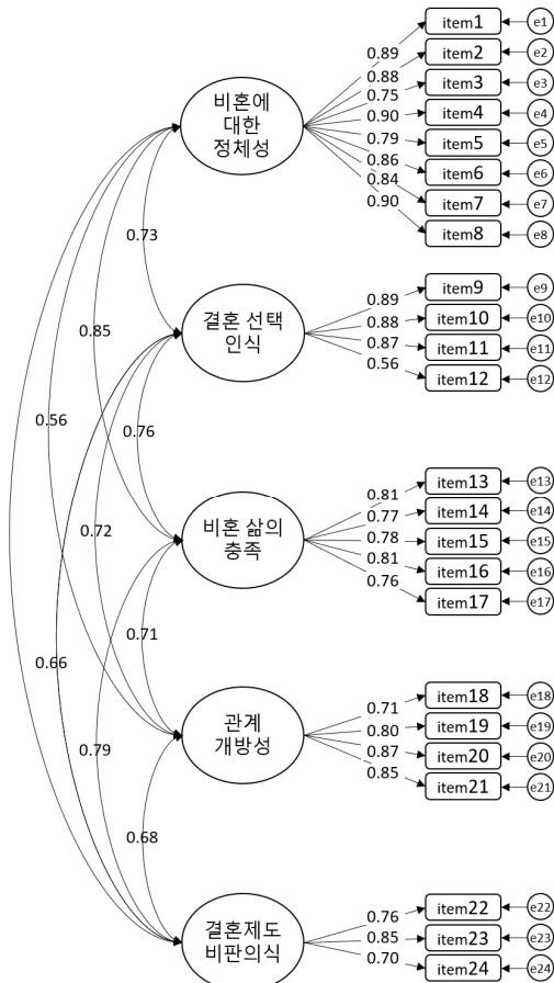
그림 1. 확인적 요인분석 표준화 추정치
