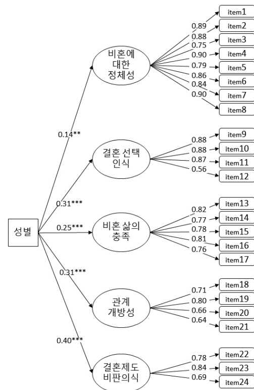
그림 2. MIMIC 분석 결과 (N = 500)
