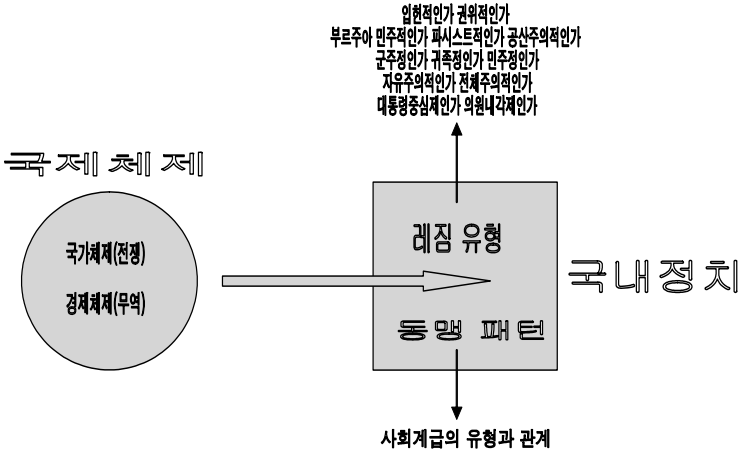
〈그림 1〉 SIR의 기본모델
