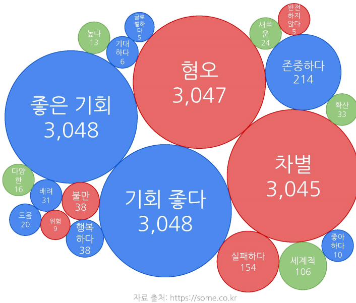
〈그림 1〉 키워드 ‘시민성’으로 드러난 한국인들의 발화 데이터(괄호 안은 빈도), (이하 그림에서 파란색은 긍정, 빨간 색은 부정, 초록색은 중립을 의미함)
