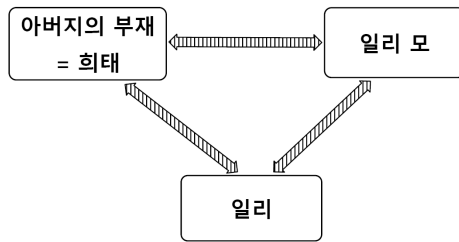
그림 2. 일리의 삼각형
