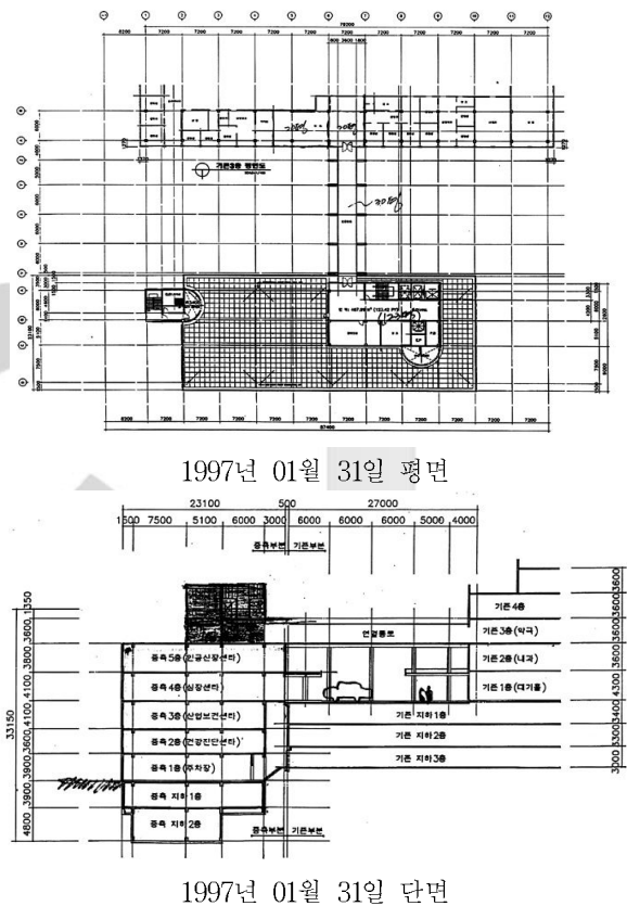
그림 11. 디자인 과정 3단계의 평면과 단면
