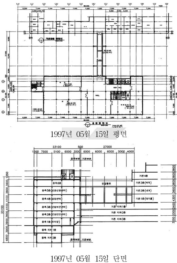
그림 12. 디자인 과정 4단계의 평면과 단면
