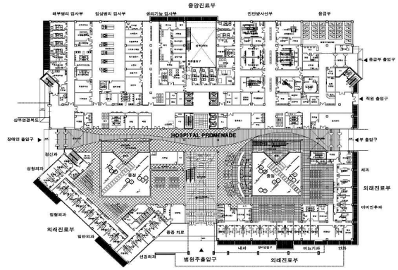
그림 15. 광주 보훈병원 1층 평면도
