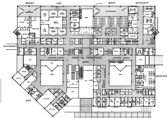
그림 16. 광주 보훈병원 2층 평면도
