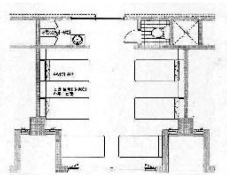
그림 18. 광주 보훈병원 다인실 평면도
