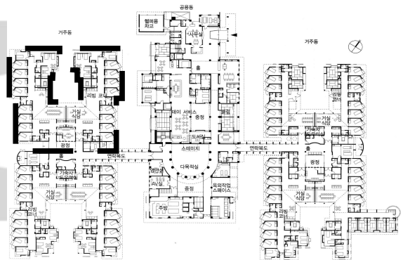
그림 7. 토카미 코우세이온 평면(특별양호노인홈, 1997)
