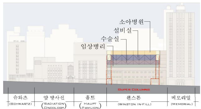
그림4. 횡단면도
