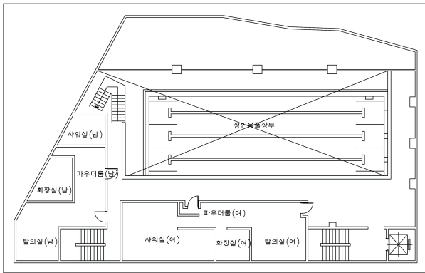
그림 12. PS11스포츠시설 평면도
