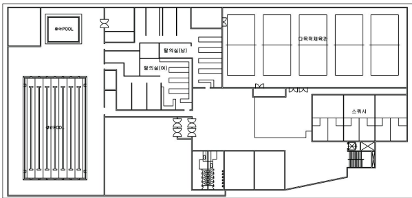
그림 4. PS01스포츠시설 평면도
