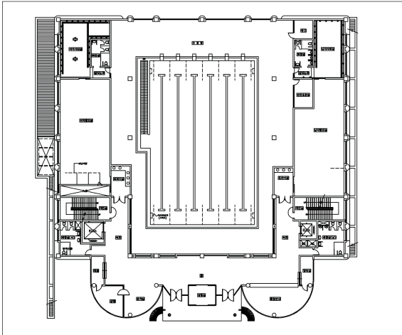
그림 16. DS02스포츠시설 평면도(1층)
