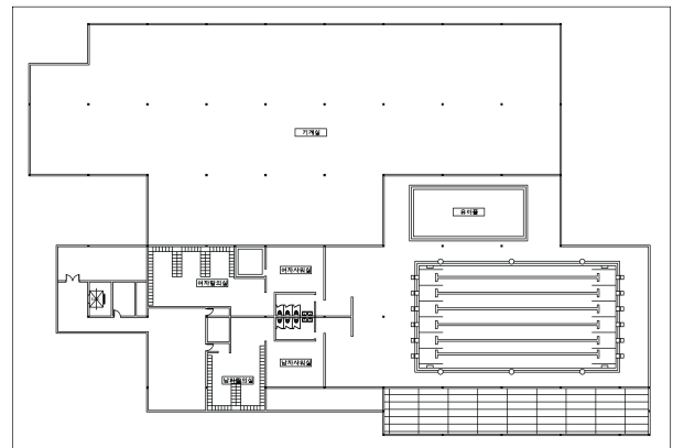
그림 10. PS04스포츠시설 평면도
