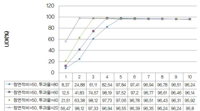
[그림 5] VT에 따른 UDI의 변화
