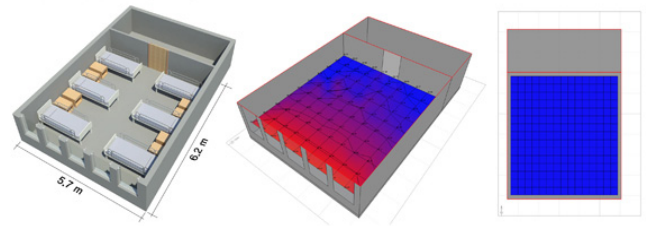
[그림 1] 시뮬레이션 유닛
