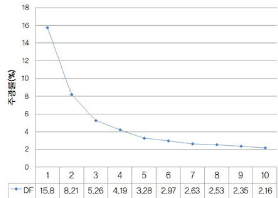
[그림 2] 창면적비 50%, 투과율 60%에서의 결과
