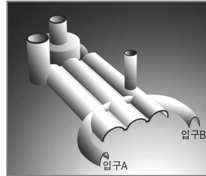
[그림 1] 용호동 '장자등 제3' 내부도(추정)
