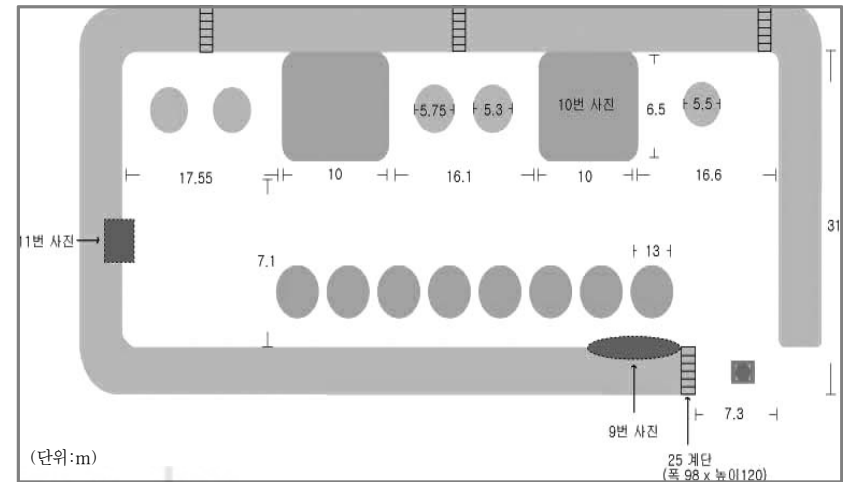
[그림 4] 외양포 포대의 전체 배치도
