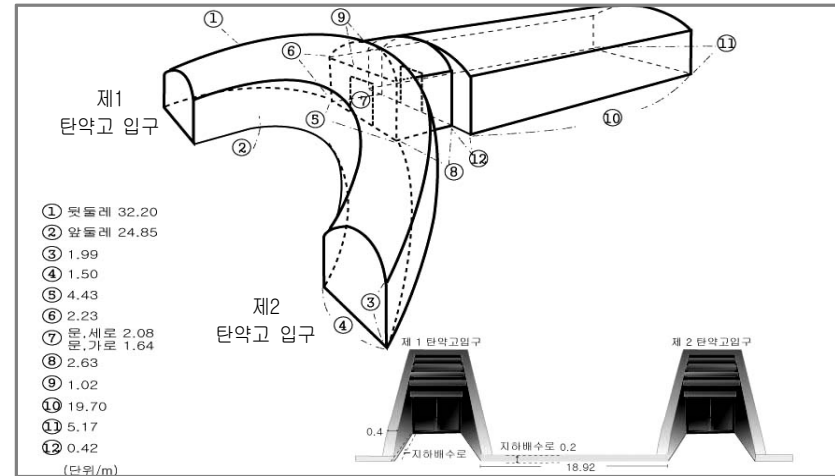
[그림 2] '장자등 제1'의 탄약고(추정)
