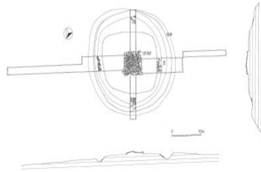
도판 1. 강릉(동해) 어달산 봉수대 실측도 * 출처 : 강릉대 박물관, 2001
