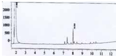
Fig. 4. GC figure of the Yinqiao San at the 5 min. after boiling it. rt 7분과 9분 사이에 많은 피크가 관찰되었으며, 11분전까지 작은 피크들이 나타나고 있다. 피크들의 크기가 전보다 많이 커졌다.
