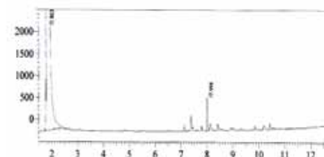
Fig. 5. GC figure of the Yinqiao San at the 10 min. after boiling it. rt 7분과 9분에서 많은 피크들이 관찰되었으며, 11분전까지 많은 작은 피크들이 나타나고 있다. 그러나 피크들의 크기가 전보다 줄어들고 있다.
