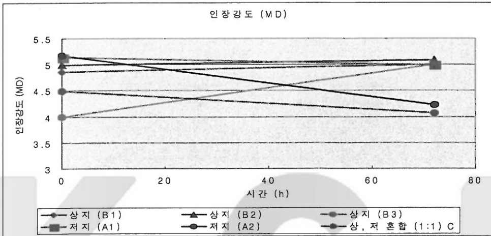
〈그림 5〉 인장강도의 변화
