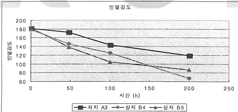
〈그림 11〉 인열강도의 변화
