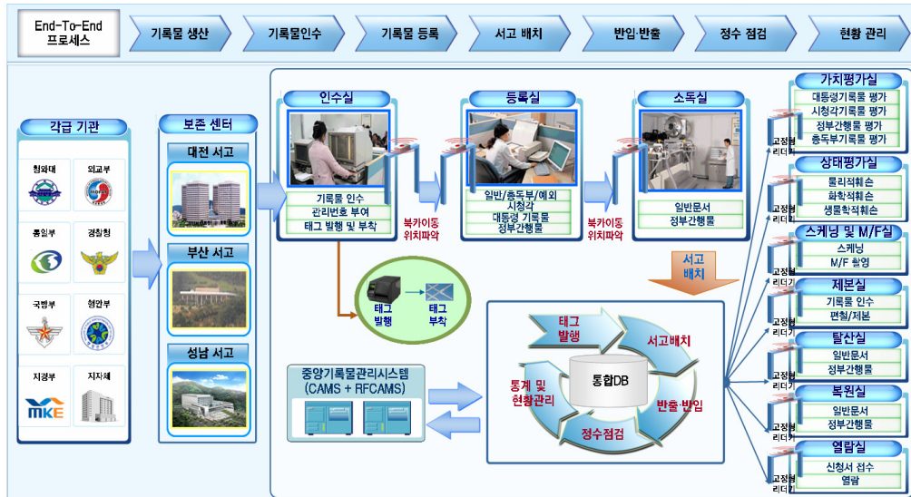
〈그림 4〉 국가기록원 RFID 시스템 구성도
