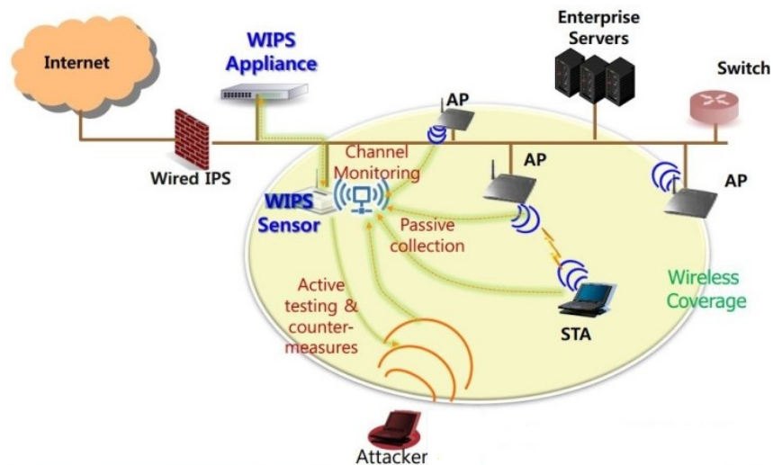
<그림 13> WIPS 구성도(예)
