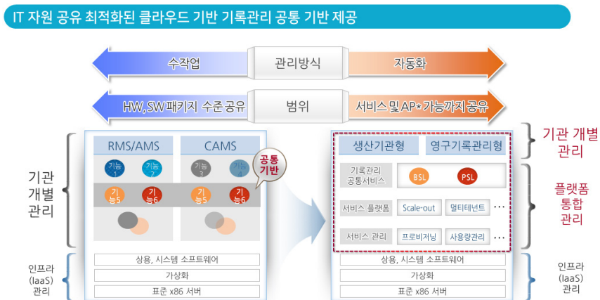
<그림 2> 클라우드 기록관리 공통 기반
