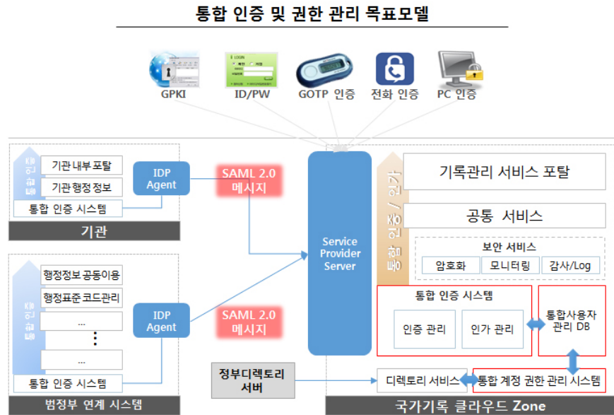
〈그림 4〉 통합 사용자 관리 구성 방안
