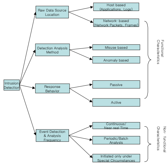
그림 3. 침입탐지유형 Fig 3. Intrusion Detection Types
