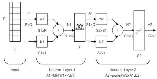
그림 4. 2 계층의 뉴로-퍼지구성도
