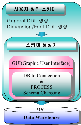
그림 2. 스키마 생성 개발 모듈 Fig. 2 Modules for developing schema generator
