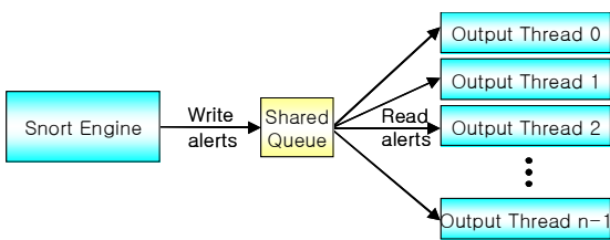
그림 2. 다중 쓰레드 모델 Figure 2. Multi-Thread Model
