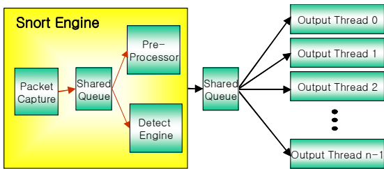
그림 4. 제안하는 네트워크 기반 침입탐지시스템 구조 Figure 4. Architecture of suggests NIDS
