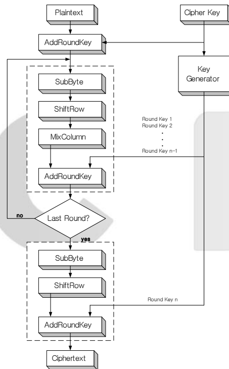
그림 1. Rijndael 암호알고리즘 Fig. 1 Rijndael cryptalgorithm
