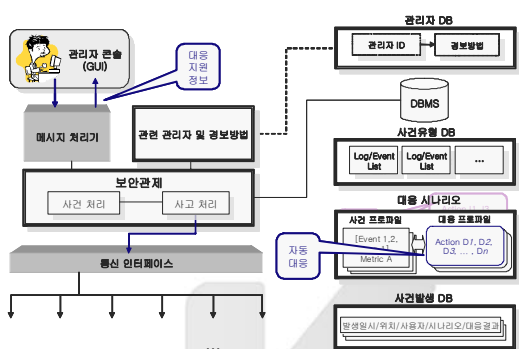
[보안대응 모듈]
