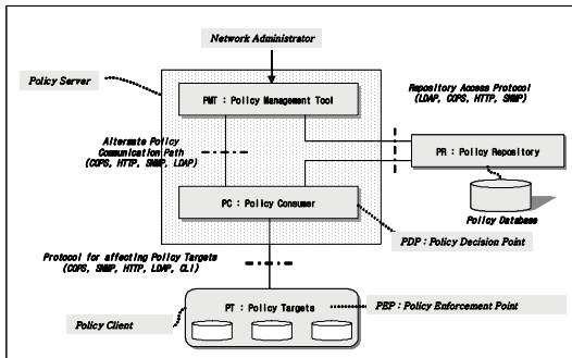
그림 1. PBNM 프레임워크 Fig. 1 PBNM Framework
