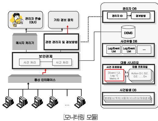
[모니터링 모듈]
