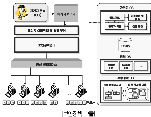
[보안정책 모듈]
