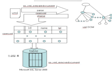
그림1. OpenXML과 2개의 시스템 프로시저
