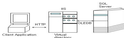
그림 2. SQL서버의 HTTP데이터 접근 구조
