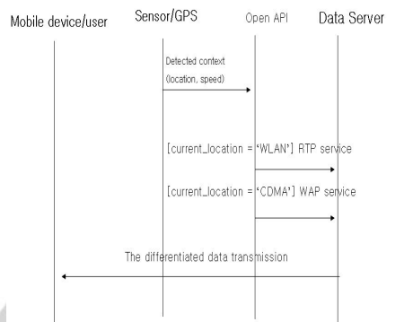
그림 3 시나리오 시퀀스 다이어그램 Fig.3 Scenario Sequence Diagram
