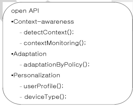
그림4. 정의된 개방형 API Fig.4 The defined open API
