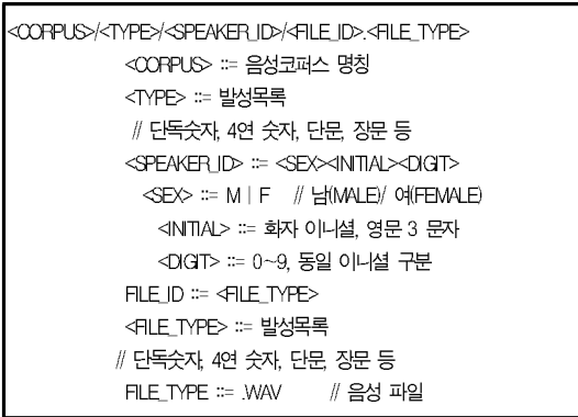
그림 2. 음성코퍼스 정보 구조 Fig 2. information structure of speech corpora
