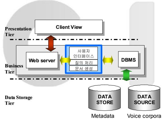
그림 4. 제안된 통합 관리 시스템 구조 Fig 4. proposed integrated management system architecture
