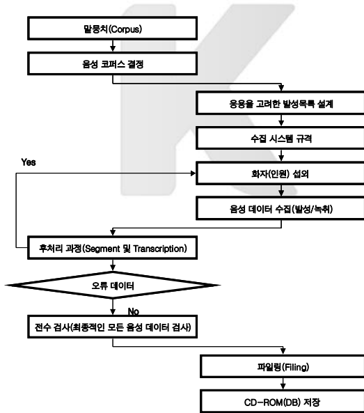
그림 3. 음성코퍼스 구축 과정 Fig 3. construction procedure of speech corpora
