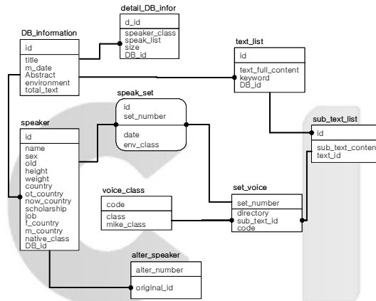
그림 5. 개체-관계 다이어그램 Fig 5. Entity Relationship Diagram
