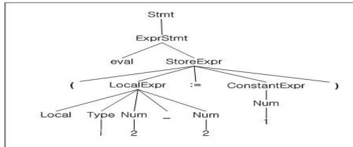
그림 6. eval(Local2.2:=1) 트리구조 Fig 6. eval(Local2.2:=1) Tree Structure
