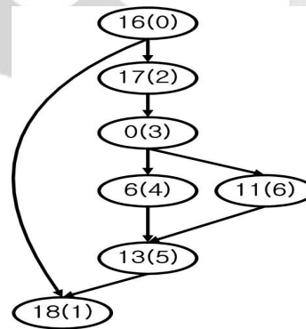
그림 8. 제어 흐름 그래프 Fig 8. Control Flow Graph
