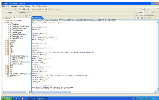
그림 13 완성된 정적 단일 배정문 형태 Fig 13. Finished Static Single Assignment Form
