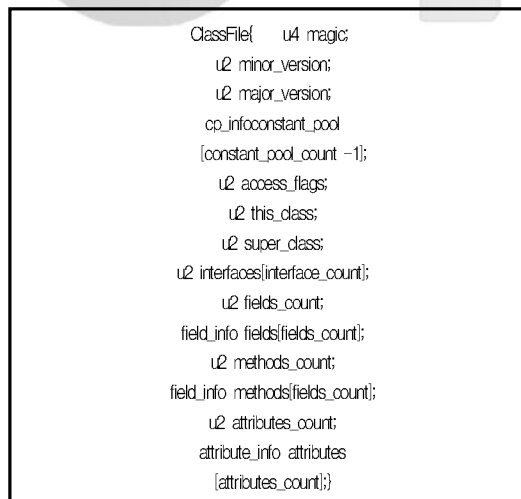
그림 1. 클래스 파일의 구조 Fig 1. Structure of Class File
