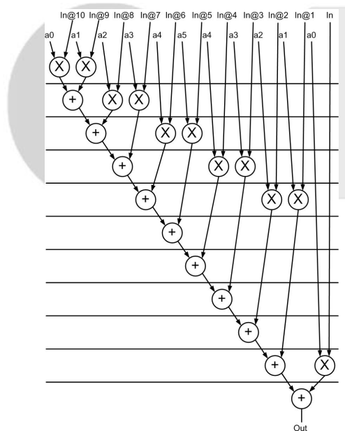
그림 1. 16 비트 FIR 필터의 스케줄링 결과 Fig. 1 Scheduling result of a 16 bit FIR filter
