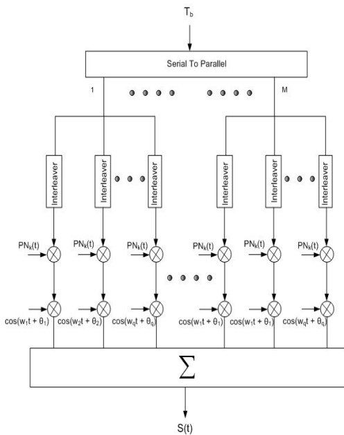
Fig.1 Multicarrier CDMA transmitter for M parallel branches with S carriers per branch 그림1. S 캐리어의 경로와 M 병렬 경로의 MC-CDMA송신기
