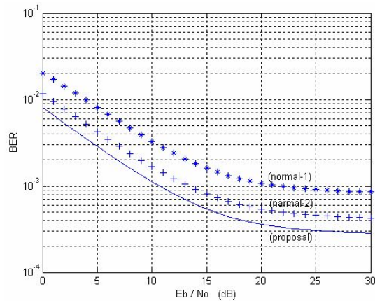
Fig 4. BER of OQPSK system 그림 4. OQPSK 시스템의 비트에러확률
