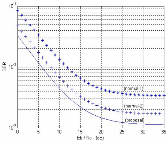
Fig 3. BER of QPSK system 그림 3. QPSK 시스템의 비트에러확률
