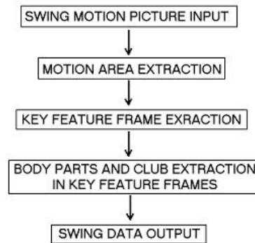
Figure 1. Flow of Feature Extraction in Swing. 그림 1. 스윙에서의 특징 추출 흐름도
