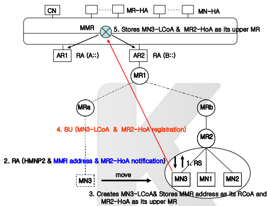
그림 4. 도메인 내 이동 노드 핸드오프 Fig 4. MN's Handoff in Intra-domain
