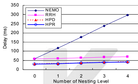
그림 6. 중점간 패킷지연 Fig 6. End-to-End Packet Delay
