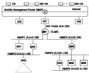
그림 1. HMNP 할당 Fig 1. HMNP assignment
