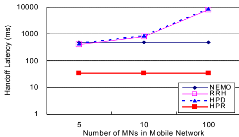
그림 8. 핸드오프 지연 Fig 8. Handoff Latency
