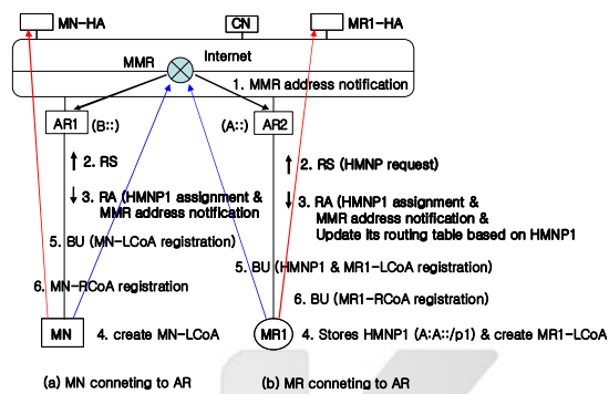
그림 2 핸드오프시 등록절차 Fig 2. Registration Processes in Handoff
