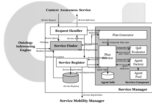
그림 6. 서비스 관리자 구성도 Fig 6. Architecture of Service Manager
