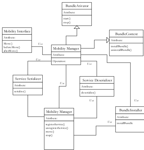
그림 9. 서비스 이동 관리자의 클래스 다이어그램 Fig 9. Class Diagram of Service Mobility Manager
