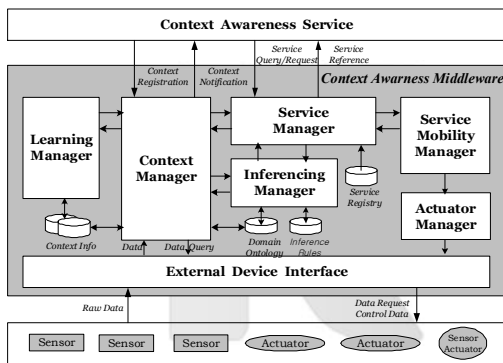
그림 5. 동적 서비스 지원 미들웨어 구성도 Fig 5. Middleware Architecture support for Dynamic Services
