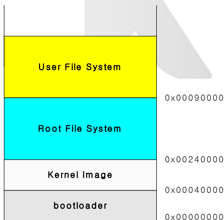
그림 4. 메모리 맵 Fig4. Memory map
