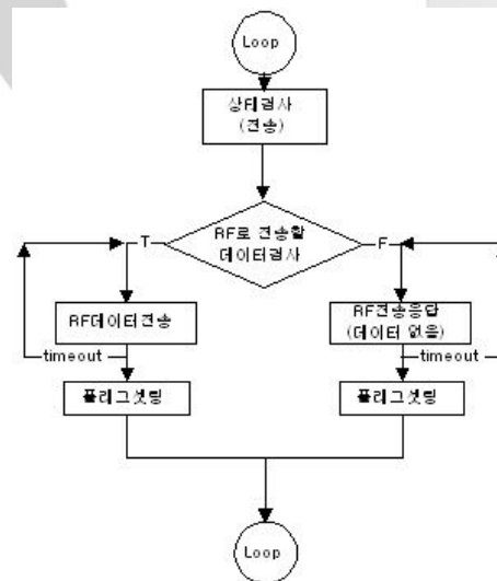
그림 3. 무선통신 플로우차트
