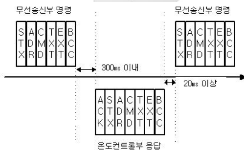
그림 2. RS485통신 구조도
