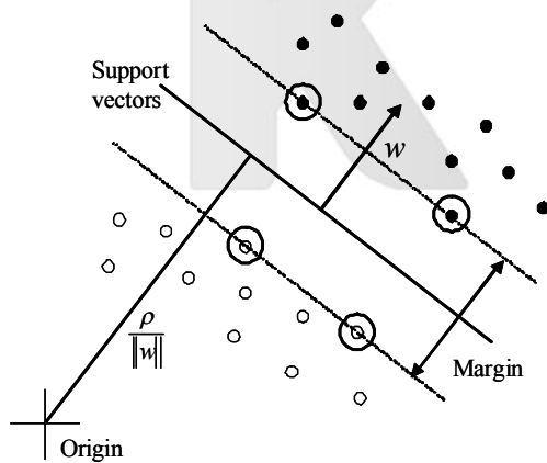
그림 1. 2차원 공간에서의 SVM의 결정경계영역 Fig 1. SVM decision boundary region of two dimensions
