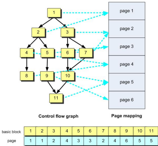
그림 3. 제어 흐름 그래프 상에서 basic block과 페이지 대응 Fig. 3. Basic block and page mapping for a control flow graph
