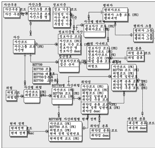
그림 15. ITRMS DB 개념설계 Fig.15 the ITRMS DB conceptual design
