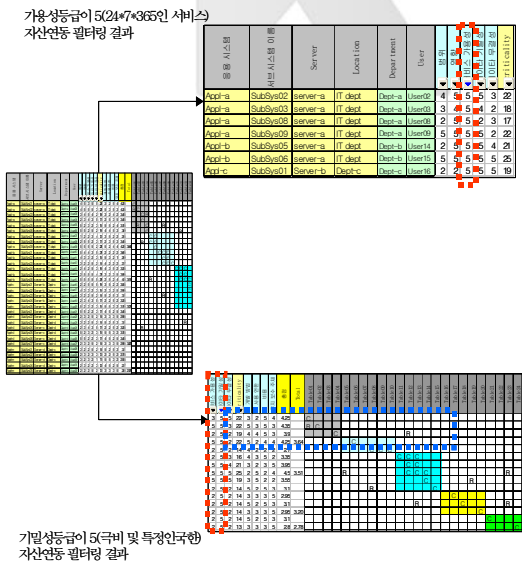
그림 8. 응용서비스 중요도 필터링 연산결과 Fig. 8 Application service important filter ring operation result
