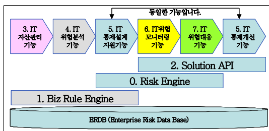
그림 2. ITRMS 기본구조 Fig. 2 the ITRMS Basic structure
