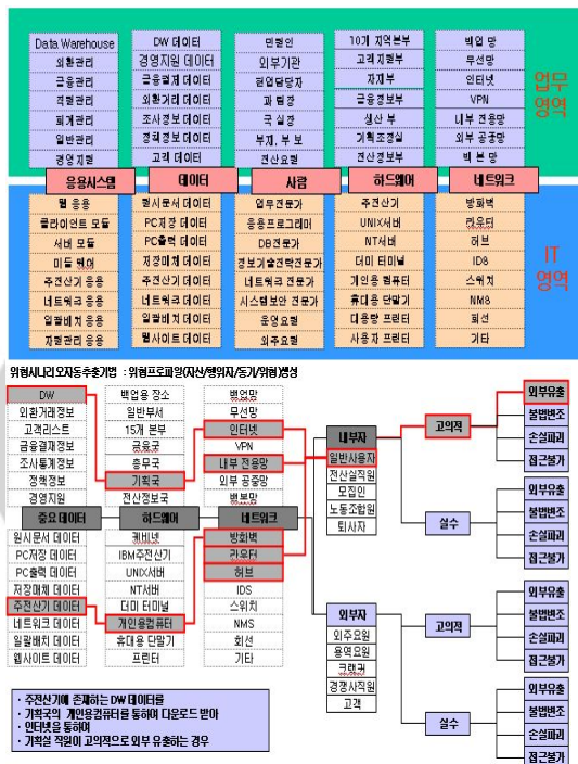
그림 9. 자산연동기법의 작동방법 Fig. 9 Operational method of the linked assets technique
