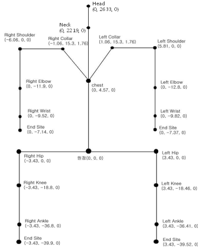
그림 7. 관절의 절대좌표 Fig. 7. Absolute Coordinate of Articulations
