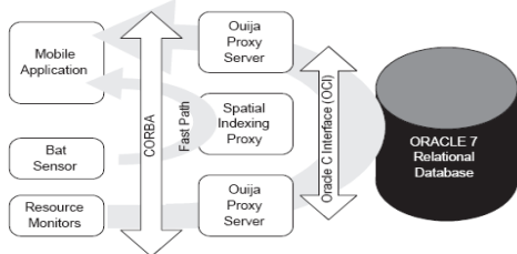
그림 5. AT&T의 시스템 구조 Fig 5. System Architecture in AT&T
