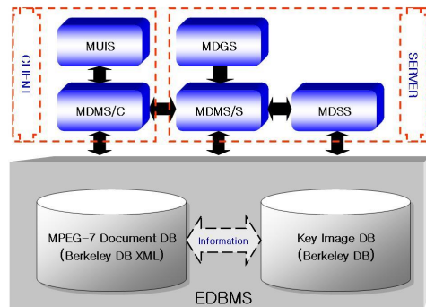
그림 2. EMDS의 시스템 구성도 Fig 2. System architecture of EMDS
