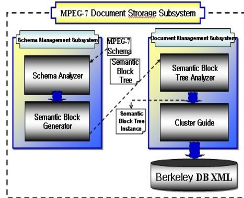
그림 6. MDSS의 구성도 Fig 6. Architecture of MDSS
