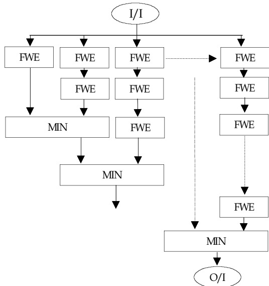
그림 5. 제안된 퍼지 웨이블릿 형태학 연산자를 적용한 DTCNN 구조 Fig. 5 DTCNN Structure with the proposal Fuzzy Wavelet Morphology Operator
