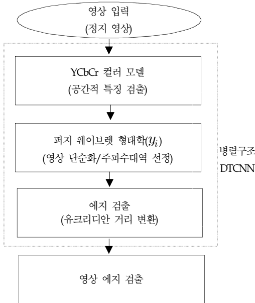
그림 4. 제안된 퍼지 웨이블릿 형태학 신경망 알고리즘 흐름도 Fig. 4 Flowchart of the proposal Fuzzy Wavelet Morphology Neural Networks Algorithm
