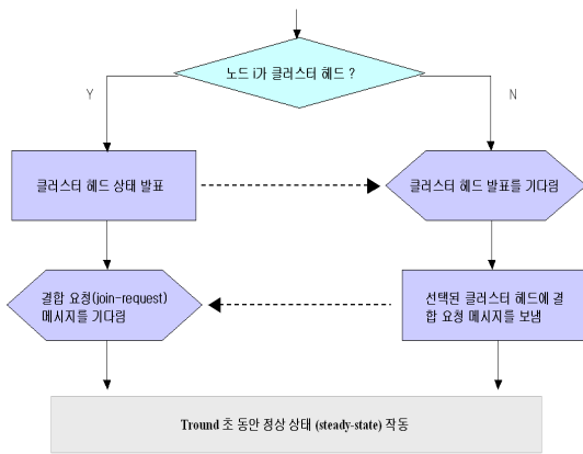
그림 1. 분산된 클러스터 형성 알고리즘 순서도 Fig 1. Flowchart of the Distributed Cluster Formation Algorithm for LEACH
