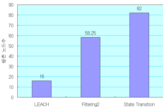
그림 10. 수행 시간이 530초일 때 생존 노드수(%) Fig 10. Number of Nodes alive at 530 Second
