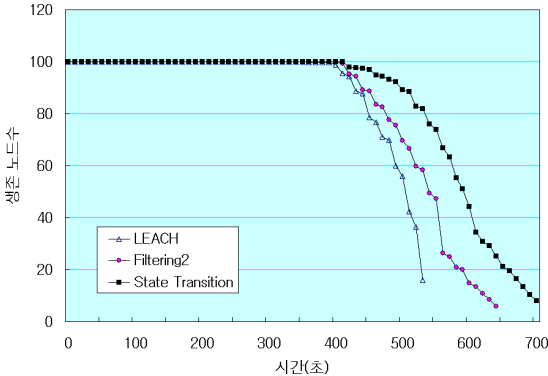
그림 9. 시간에 따른 생존 노드수 Fig 9. Number of Nodes alive over Time
