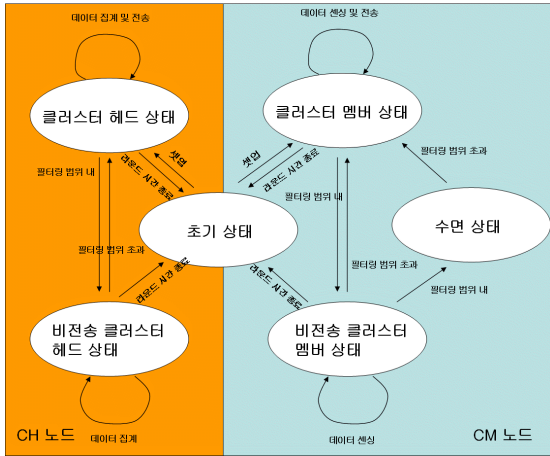
그림 3. 노드의 클러스터 상태 전이 Fig 3. Cluster State Transition of Sensor Node
