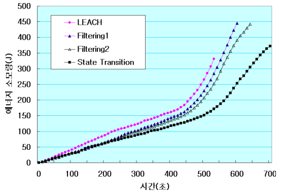
그림 5. 시간에 따른 에너지 소모량 Fig 5. Amount of Energy Dissipation over Time
