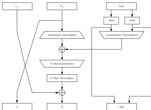
그림 3. DES의 한 라운드(round) Fig 3. One round of DES
