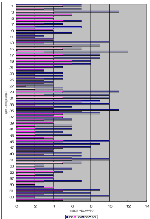
그림 9. 평문 한 비트의 변화에 따른 암호문 비트의 변화량 비교 Fig 9. Comparison of change of encryption text bits by plaintext change
