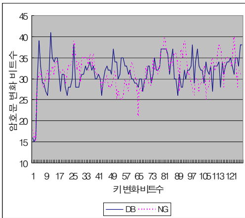
그림 12. 키 비트의 변화에 따른 암호문 비트의 변화량 비교 Fig 12. Comparison of change of encryption text bits by key bit change
