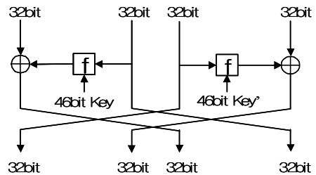
그림 4. NG-DES의 한 라운드 Fig 4. One round of NG-DES
