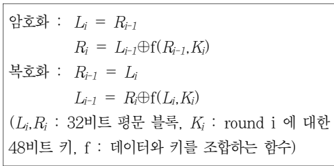
그림 2. DES의 암호화와 복호화 공식 Fig 2. Encryption and decryption formula of DES
