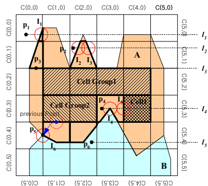
그림 9. 공간 영역 A의 셀과 단방향 직선 l과의 교차에 따른 포함 관계 Fig.9. Inclusion Relationship on the Intersection Cells of Area A with Line l
