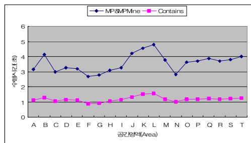
그림 14. 공간영역으로의 일반화 수행에 따른 성능비교 Fig.14. Performance Comparison to perform Generalization into Spatial Region
