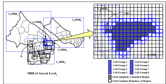
그림 6. L 3 의 MBR에 대한 Grid 분할 Fig.6. The Grid Division against MBR of the L 3
