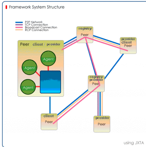
그림 6. 프레임워크 시스템 구조 Fig 6. Framework System Structure
