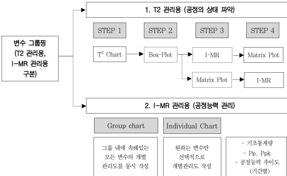
그림 1. 조기경보시스템 흐름도 Fig 1. Flow chart of early warning system
