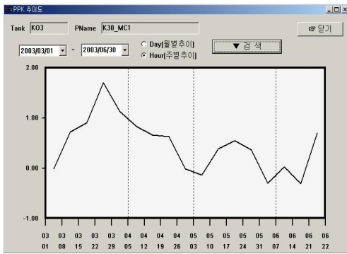
그림 6. 공정능력지수 추이 Fig 6. PCI(PPK) Trend diagram
