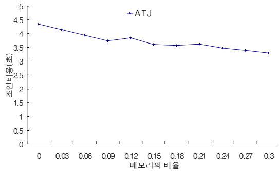
그림 3. 메모리 용량변화에 따른 성능 변화 Fig. 3 Effect fo memory capacity on ATJ
